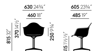
Eames Plastic Armchair RE DAL
