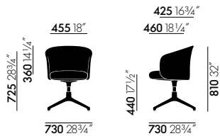
Mikado Armchair, viersteronderstel
